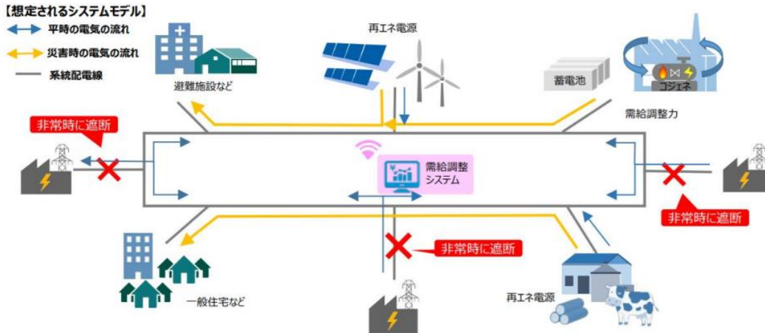
地域マイクログリッドの概要図(資源エネルギー庁「地域マイクログリッド構築のてびき」より)
